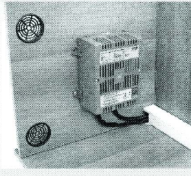
Fig.2 - INSTALLAZIONE VERTICALE
