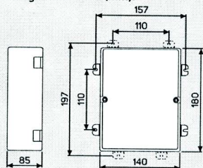
Abbildung 1 - ABMAßE (mm):
