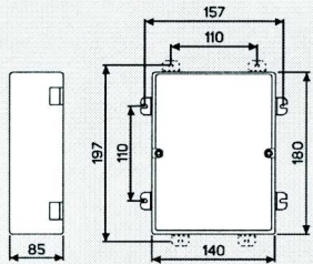
Fig.1 - DIMENSIONI (mm):
